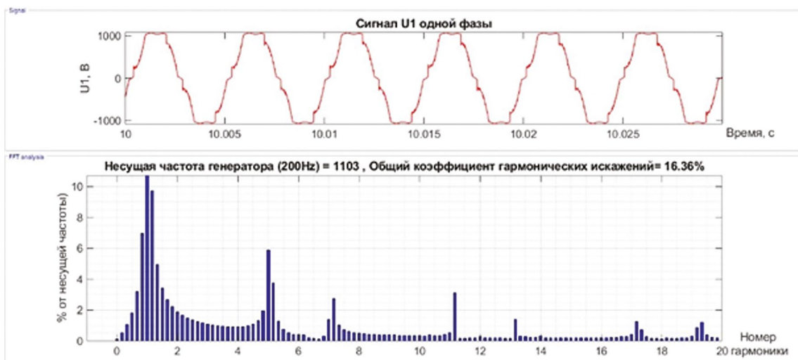
Рис. 2. Гармонический состав на статоре генератора с использованием активного выпрямителя
