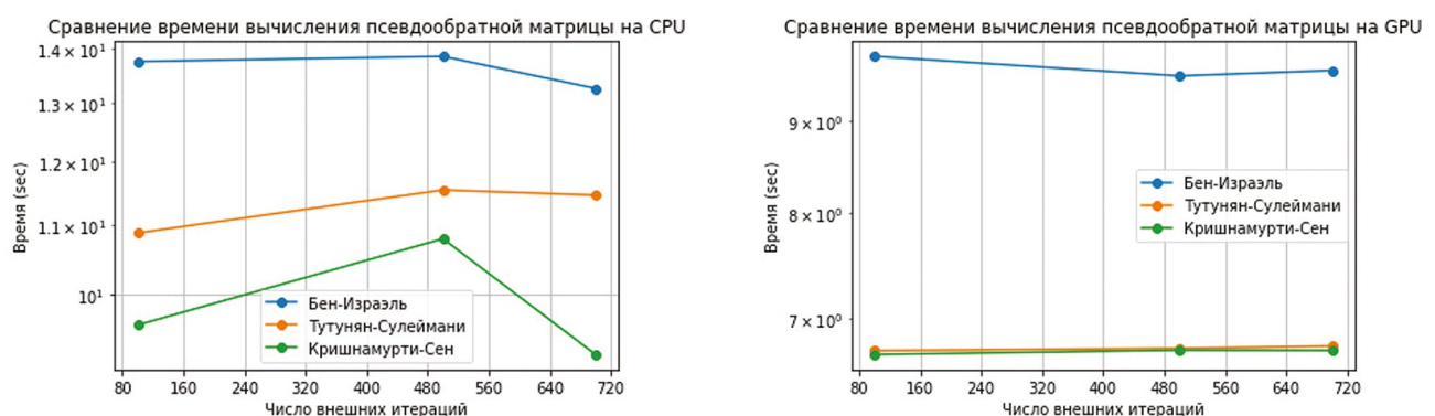
Рис. 1. Тестовая задача с матрицей A^{4096 \times 4096}
